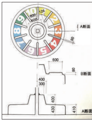
ルーレットベンチの図面
